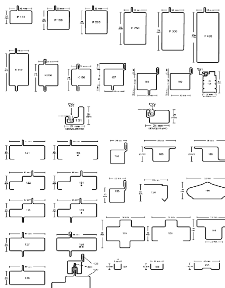
PERFIL TUBULAR
